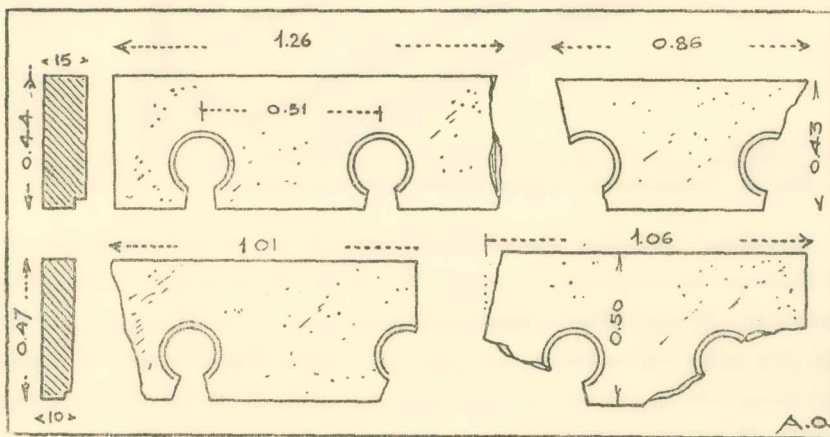
Εἰκ. 5. Μαρμαρίναι πλάκες μετ' ὀπῶν ἀφοδεύσεως.
