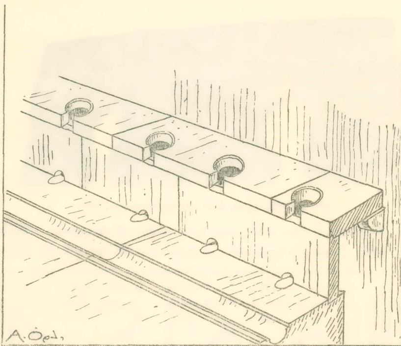
Εἰκ. 6. Ἀναπαράστασις τμήματος τῶν διατηρήτων καθισμάτων τοῦ ἀφοδευτηρίου.
