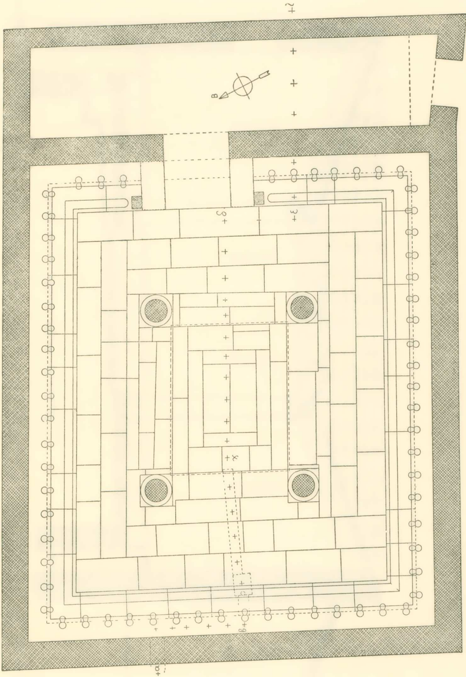
Είχ. 2.—'Αναπαράσταση τῆς κατόψεως τῶν ἀφροδευτηρίων.
