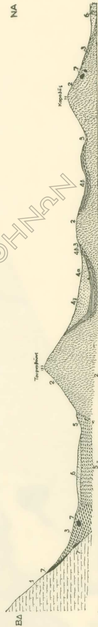
Τομή 2.— 1. Τριαδικός άσβεστολίθος.— 2. Συμπαγείς Κρητιδικοί άσβεστολίθοι.— 3. Πλακώδεις Κρητιδικοί άσβεστολίθοι και μάργαι.— 4α λατυποπαγές υπό τὸ σύστημα των σχιστολίθων των Άθηνών.— 4β Κατωτάτη βαθμὶς του συστήματος των σχιστολίθων των Άθηνών εκ μαργών και άσβεστολίθων.— 4γ Άργιλικοί σχιστολίθοι και ψαμίται του συστήματος των Άθην. σχιστολίθων.— 5. Νεογενή.— 6. Τεταρτογενή.— 7. Περιδοτίται.
