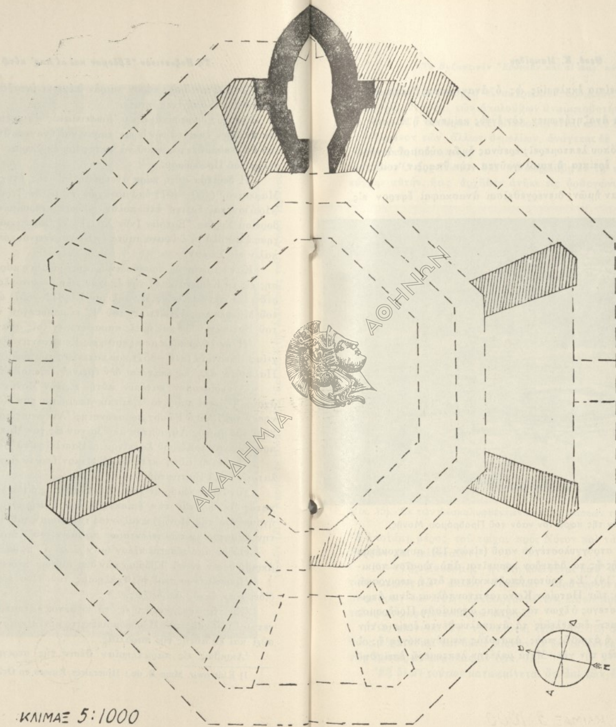
Εικών 13). Κάτοψις τοῦ ναοῦ Ἀΐροδρόμου κατόπιν τῶν ἀνασκαφῶν.
