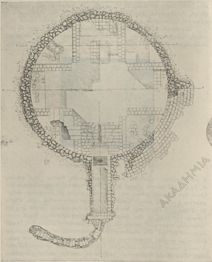
(Εἰκὼν 19). Κάτοψις τοῦ κοιμητηρίου καὶ τμήματος τῆς στέγης πρὸς τὰ δεξιά.
