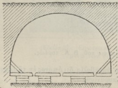
(Σχεδ. Γ). Τομὴ καὶ διάτρητον δάπεδον τῆς κρύπτης Ἁγ. Παντελεή- μονος Ἄνω Βοσπόρου.
